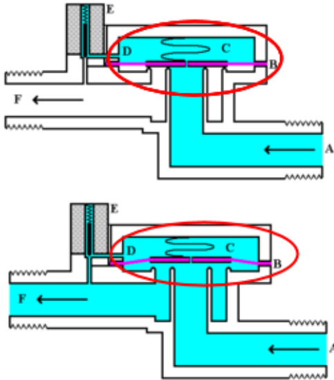
Schéma de fonctionnement
